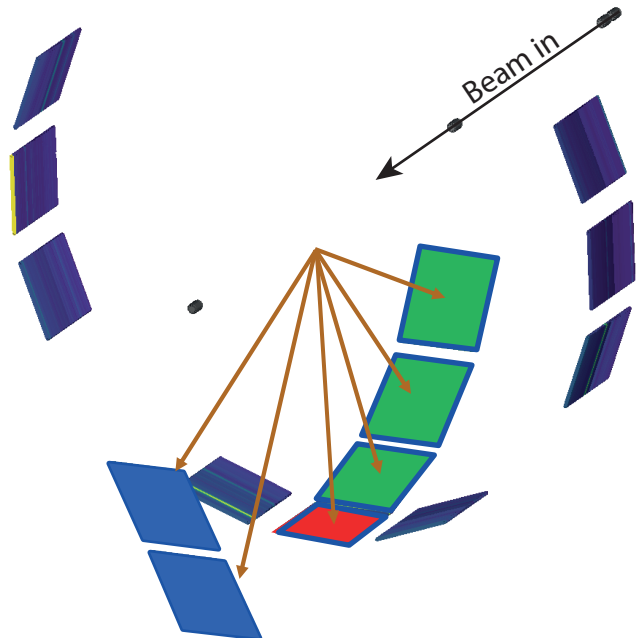
'Longitudinal' scattering geometry
